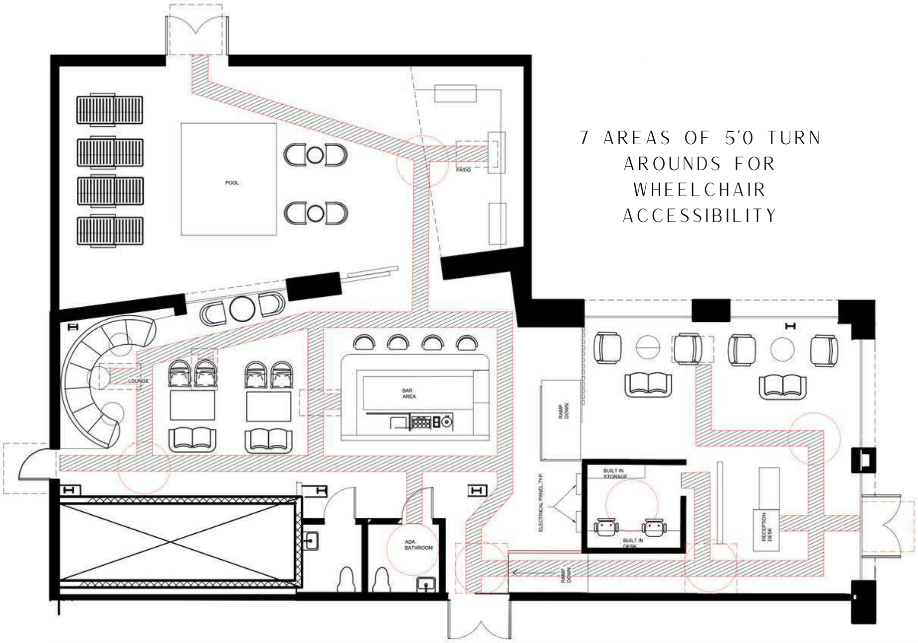
ADA EGRESS PLAN AUTO CAD
